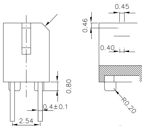
A-A' Section
